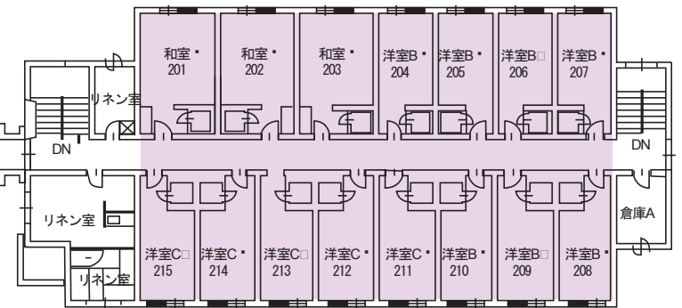
附属宿泊施設2階 平面図
